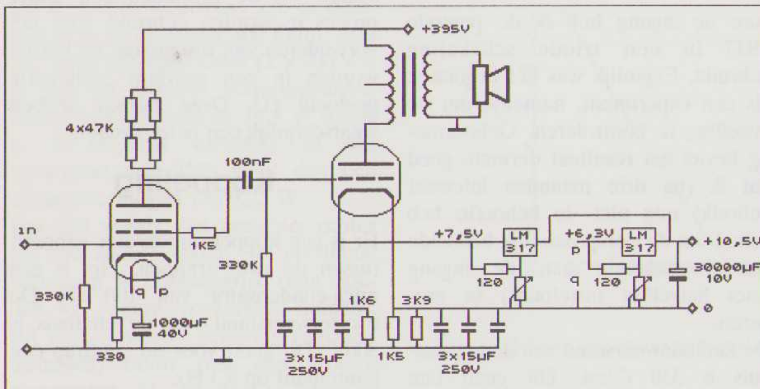
Fig. 1a. De schakeling van de versterker
